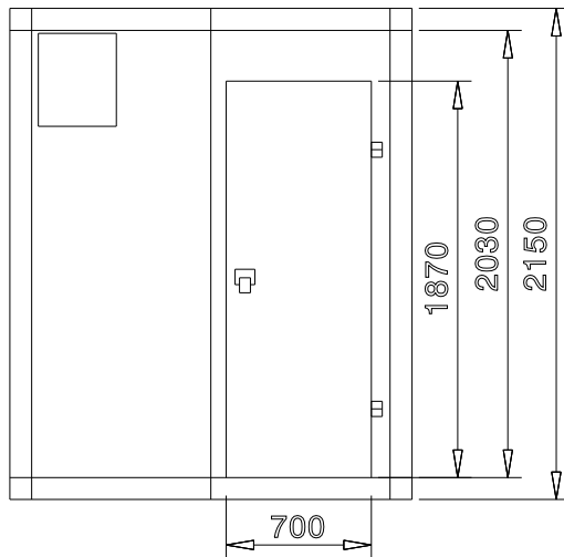
Zij aanzicht
