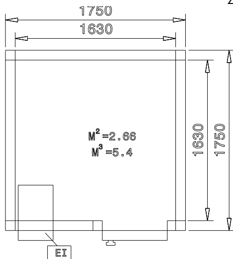
Boven aanzicht
